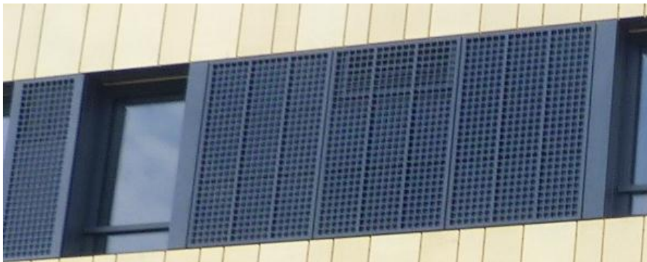
Abbildung 1: Fine Energy Modul Fassade mit vorgehängter Metallkonstruktion (Annen & Schibig AG, Muotastrasse 63, 6438 Ibach)
